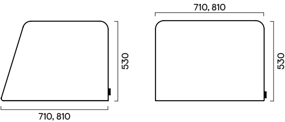
Mampara separadora de bancos NOVA
